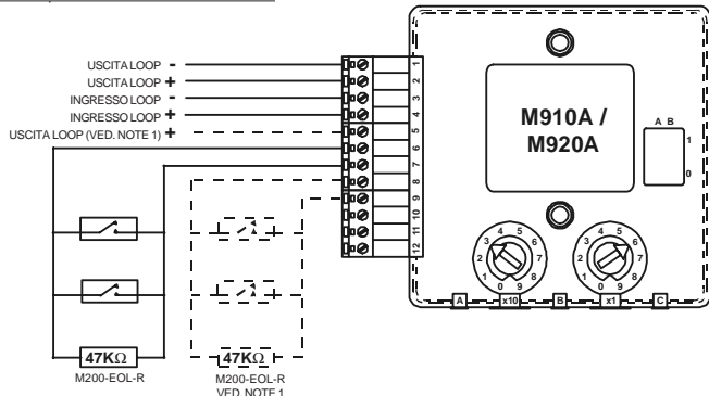
FIGURA 3: CABLAGGIO DEL MODULO A INGRESSO SINGOLO M910A E A INGRESSO DOPPIO M920A
