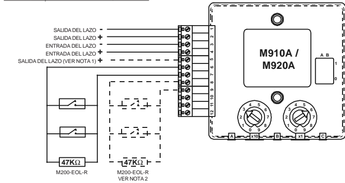
FIGURE 3: CONEXIONES DE LOS MÓDULOS M910A DE ENTRADA ÚNICA Y M920A DE ENTRADA DOBLE
