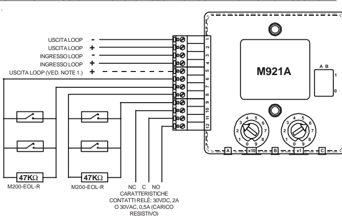
FIGURA 4: CABLAGGIO DEL MODULO A USCITA SINGOLA E DOPPIO INGRESSO M921A
