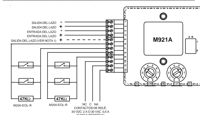
FIGURA 4: CONEXIONES DEL MÓDULO DE ENTRADA DOBLE Y SALIDA ÚNICA M921A
