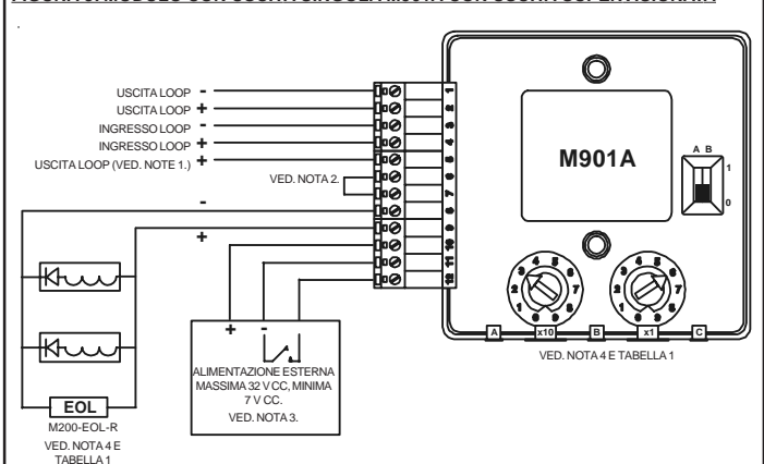
FIGURA 3: MODULO CON USCITA SINGOLA M901A CON USCITA SUPERVISIONATA
