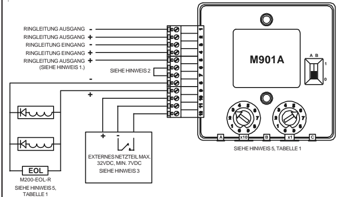
ABBILDUNG 3: M901A STEUERMODUL MIT EINEM ÜBERWACHBAREM AUSGANG
