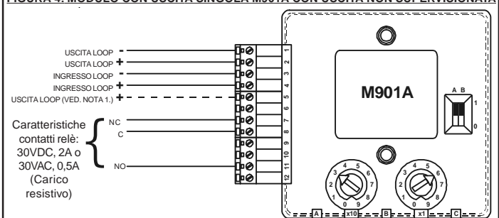
FIGURA 4: MODULO CON USCITA SINGOLA M901A CON USCITA NON SUPERVISIONATA
