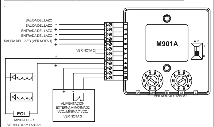
FIGURA 3: MÓDULO DE SALIDA ÚNICA M901A CON SALIDA SUPERVISADA
