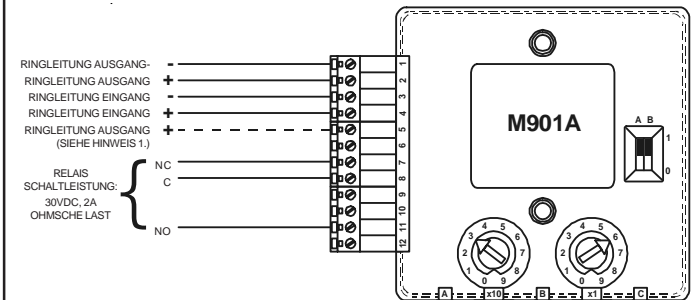
FIGURE 4: M901A STEUERMODUL MIT EINEM NICHT ÜBERWACHEM AUSGANG
