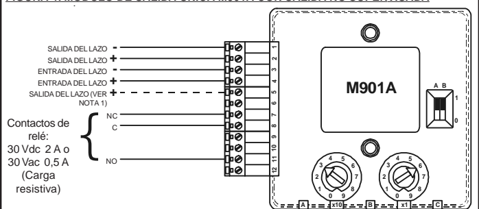
FIGURA 4: MÓDULO DE SALIDA ÚNICA M901A CON SALIDA NO SUPERVISADA
