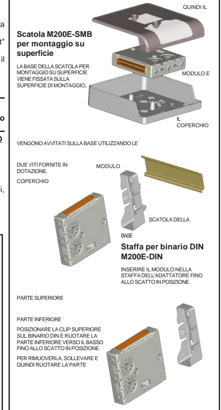
FIGURA 1: METODI DI MONTAGGIO DEL MODULO
